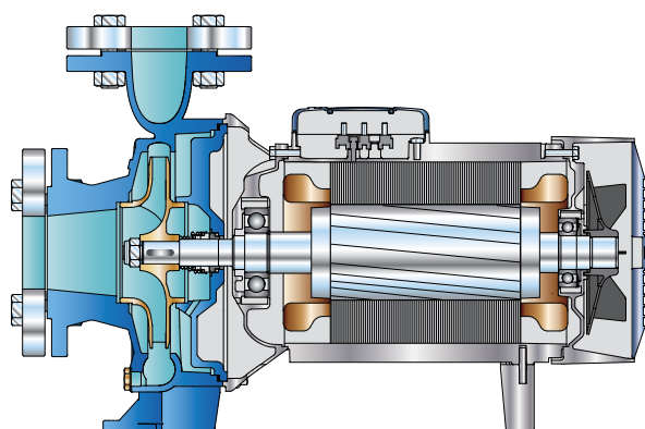
Versione trifase
