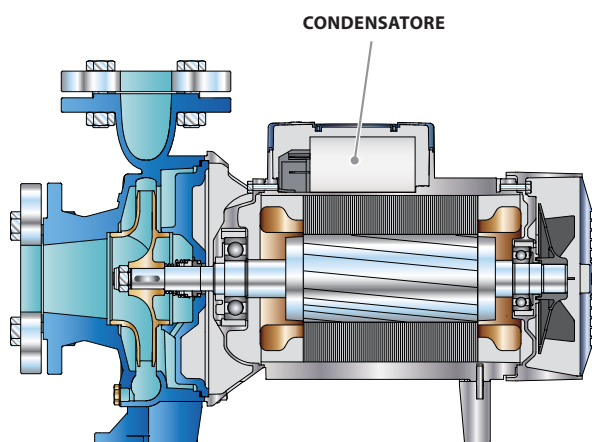
Versione monofase
