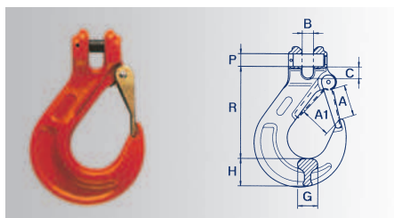
Gancio a forcella
