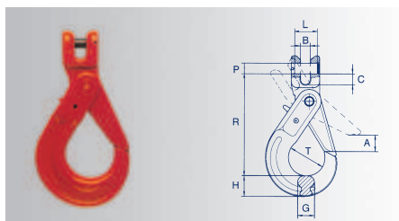
Gancio di sicurezza a forcella
