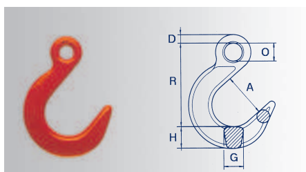
Gancio per fonderia
