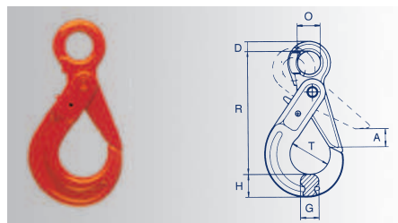
Gancio di sicurezza ad occhio
